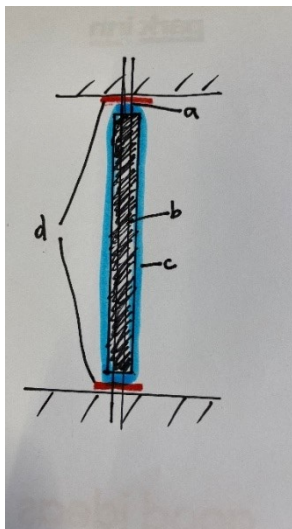
Billede 4—22. Skitse af røret og princippet af fjernelsesproces. a-uisolaret del af røret, b-asbestholdig isolering, c-plastikfolie forsegling, d-skæringspunkter.
